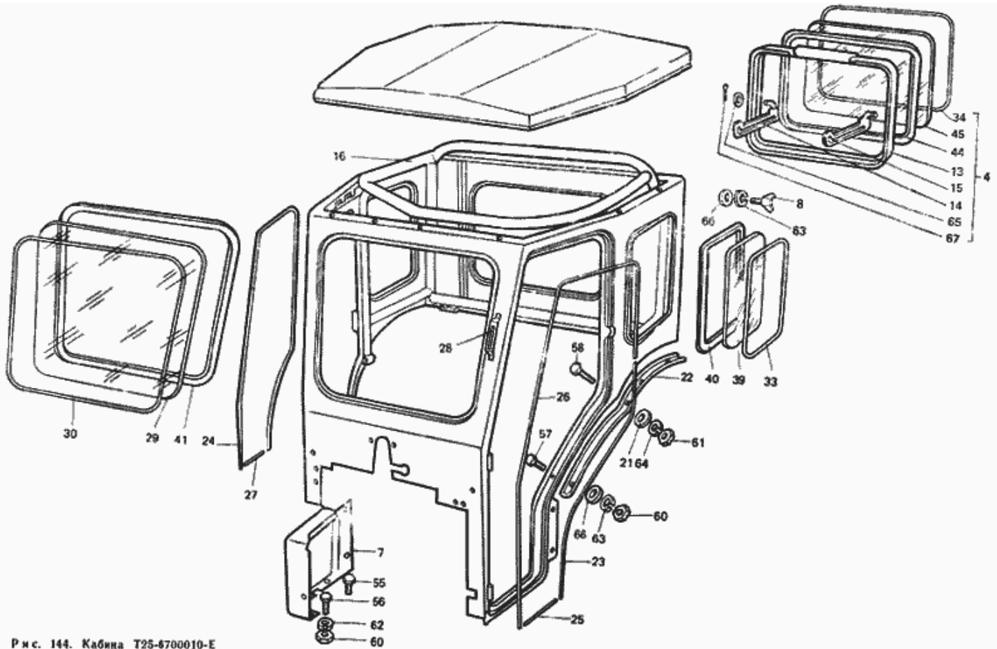
Рис. 144. Кабина Т25-6700010-Е
